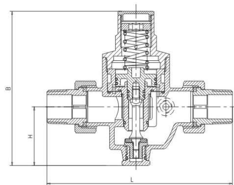
Fig: MV80-116(DN15-DN25)
