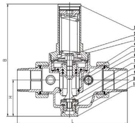
Fig: MV80-116(DN32-DN100)
